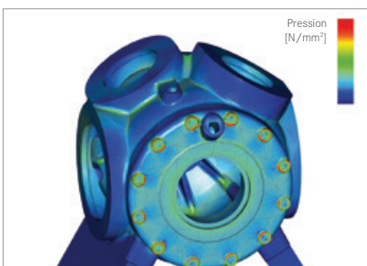
Partie supérieure droite : Piston Centre gauche : Intérieur de cylindre affiné Partie inférieure gauche : Calcul FEM pour le carter moteur Droite : bloc compresseur BK 26
